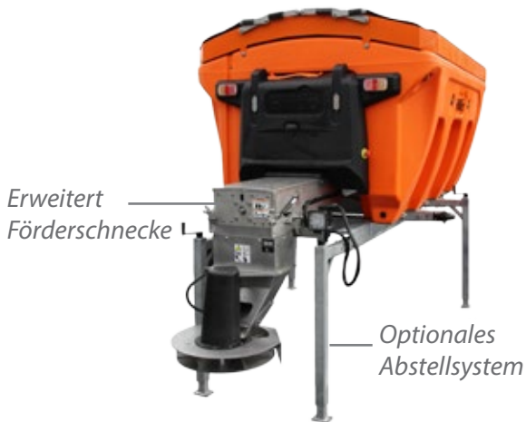
IceStriker™ 2100 in der optionalen Farbe Orange
